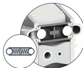
弹簧承载的球阀
